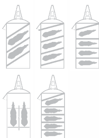
Disposition typique des bat-flancs dans le HB610
